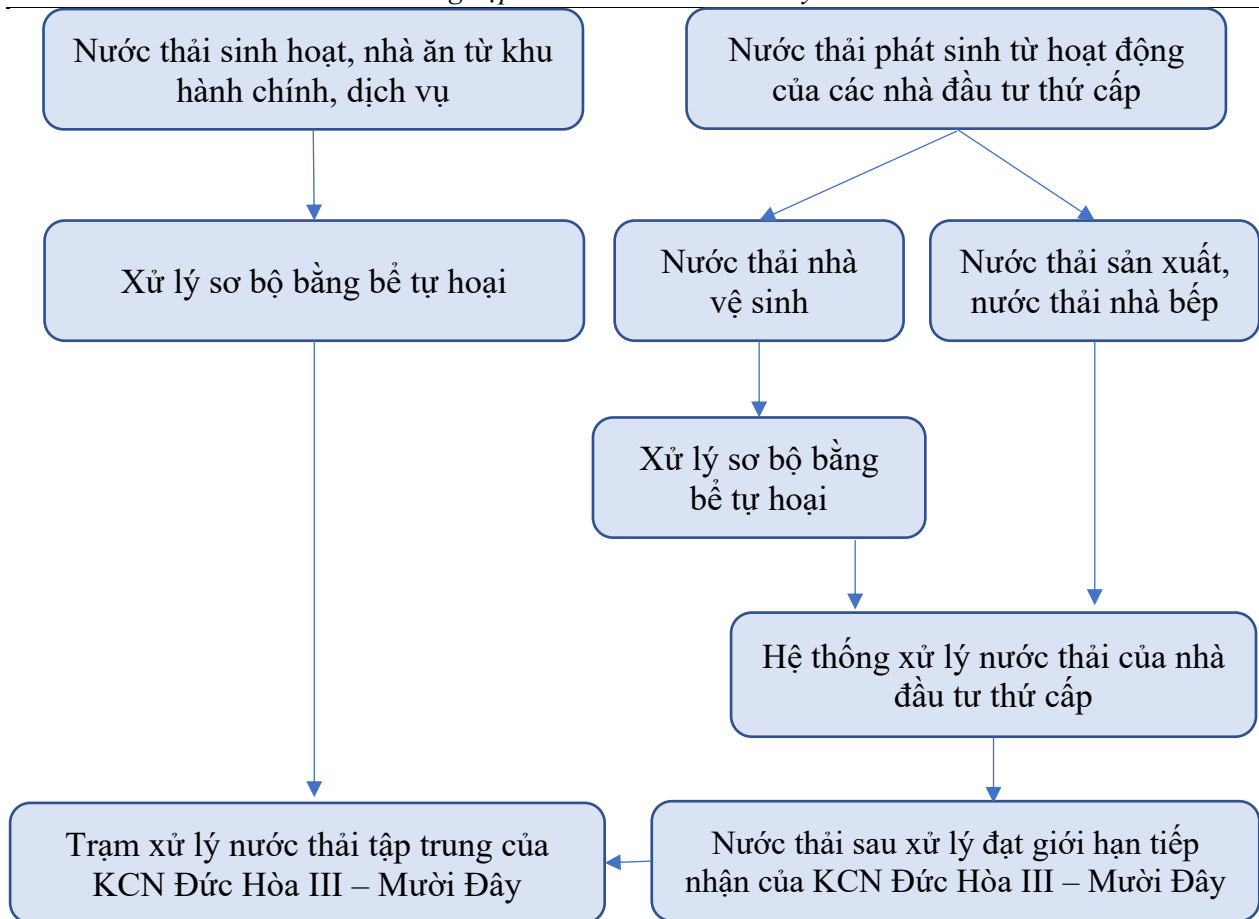
Hình 3.2. Quy trình thu gom và xử lý nước thải của KCN Đức Hòa III-Mười Bảy
