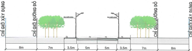
MẶT CẮT 4-4
