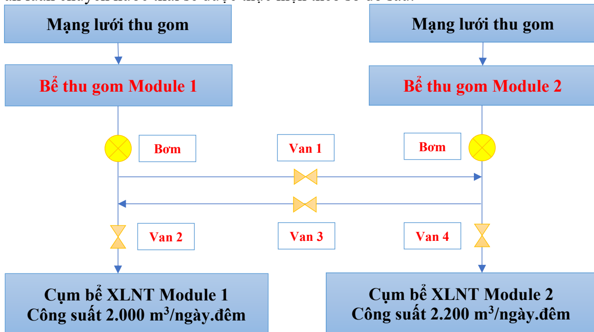
Hình 3.5. Sơ đồ quay vòng nước thải từ Module gặp sự cố về Module còn lại của Trạm XLNT
