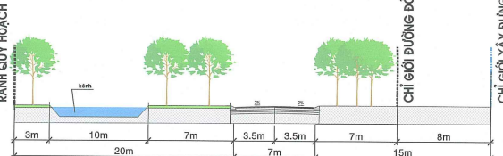
MẶT CẮT 6-6
