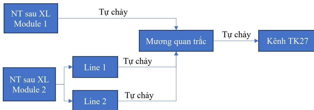
Hình 3.3. Biện pháp xả nước thải của trạm XLNTTT
