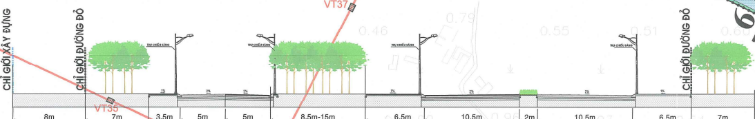
MẶT CẮT 1-1
