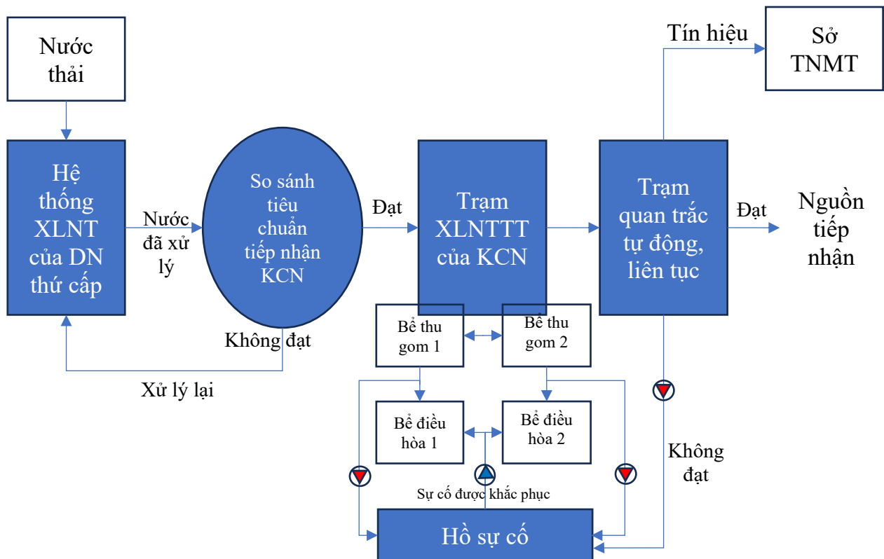
Hình 3.1. Sơ đồ kiểm soát nước thải của KCN Đức Hòa III-Mười Bảy Quy trình thu gom và xử lý nước thải của KCN Đức Hòa III-Mười Bảy như sau:
