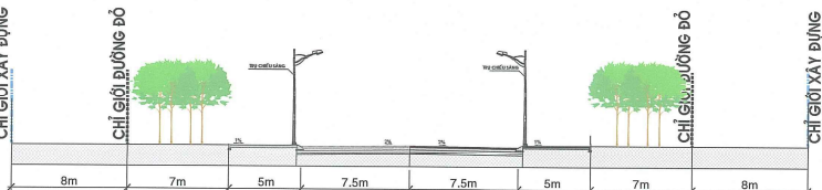
MẶT CẮT 5-5
