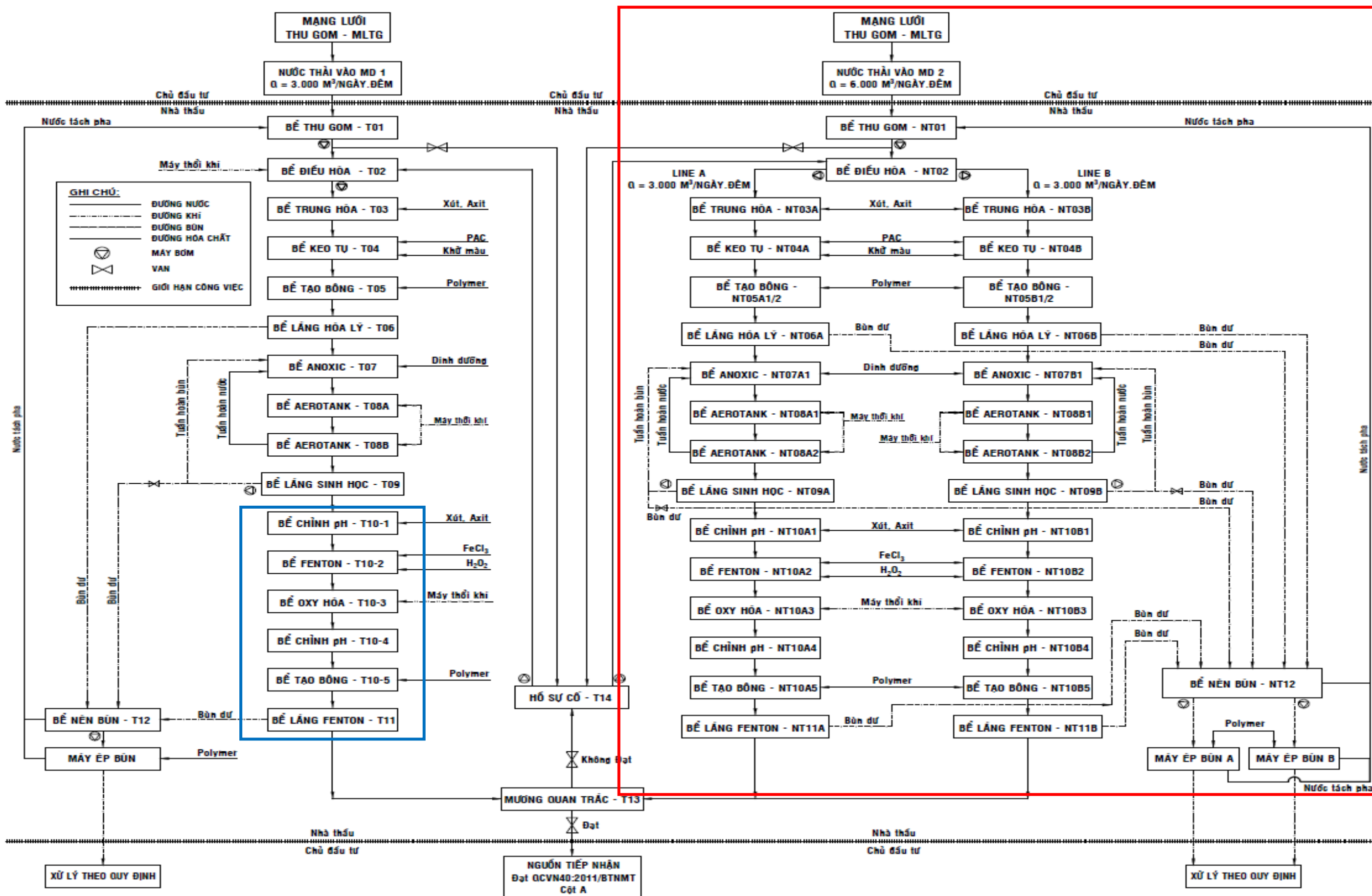
Hình 3.4. Sơ đồ công nghệ trạm xử lý nước thải tập trung
