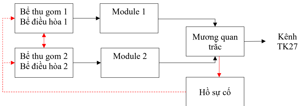
Hình 3.6. Sơ đồ ứng phó sự cố bằng sự kết hợp hồ sự cố và quay vòng nước thải từ Module gặp sự cố về Module còn lại của Trạm XLNT
